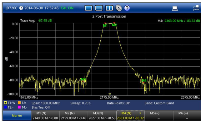
Übertragungsparameter an 2 Ports
