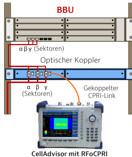
Abbildung 23: BBU mit Sendesektoren ( \alpha , \beta , \gamma ) und optischem Koppler
