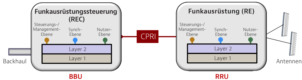
Abbildung 9: Ebenen der Protokoll Daten
