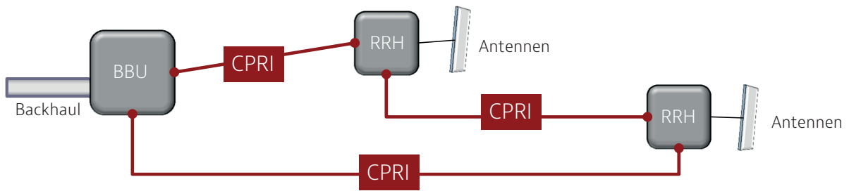
Abbildung 5: Ring-Topologie
