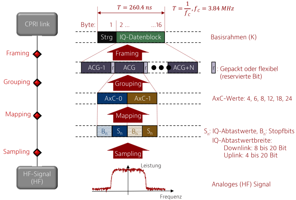
Abbildung 13: Aufbau des CPRI-Rahmens
