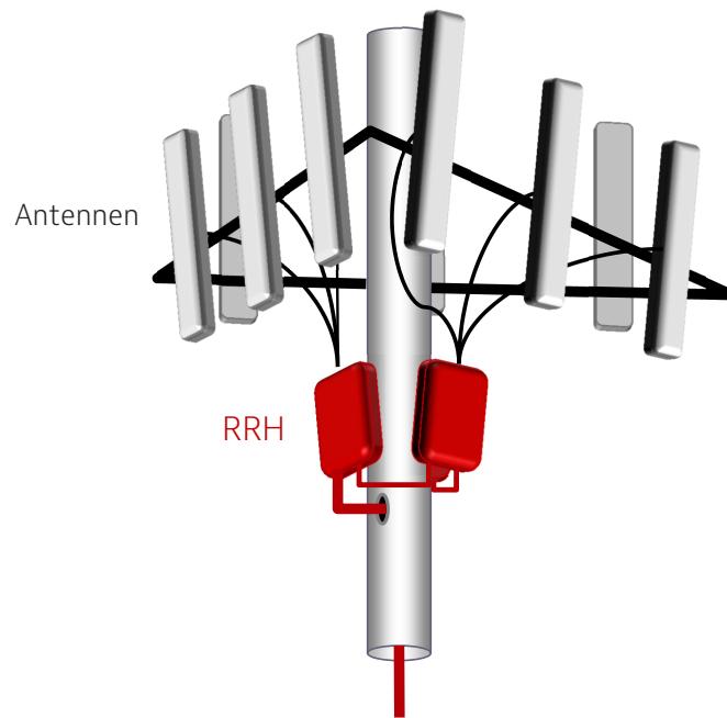
Abbildung 8: Makrozelle mit RRH in Daisy-Chain-Topologie
