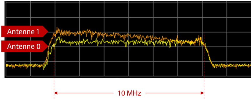
Abbildung 24: RToFoCPRI-Spektrogramm-Analyse an einem LTE-Uplink bei 10 MHz MIMO mit Intermodulationen
