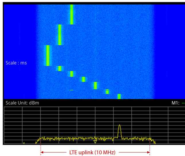
Abbildung 25: RToFoCPRI-Spektrogramm mit sporadischen Interferenzen
