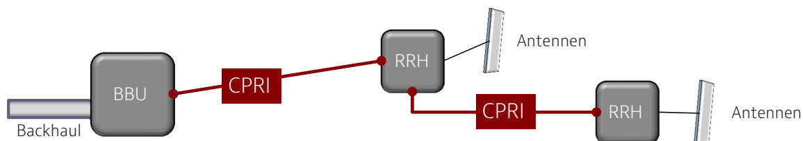
Abbildung 3: Ketten-Topologie
