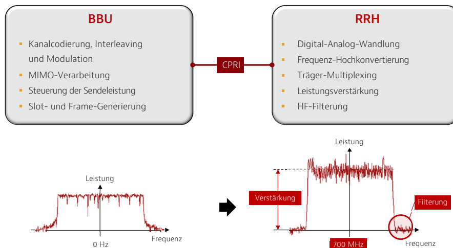
Abbildung 10: Sendefunktionen von BBU und RRH (Downlink)
