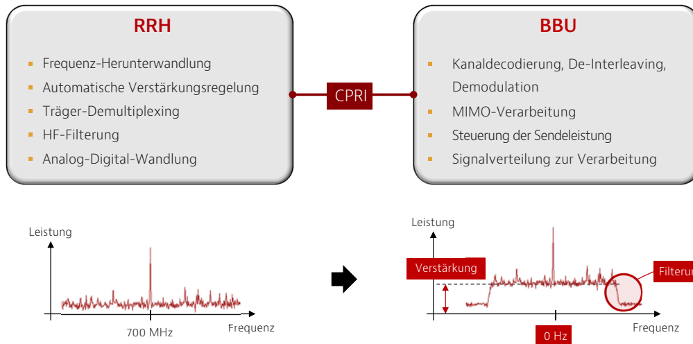
Abbildung 11: Empfangsfunktionen von BBU und RRH (Uplink)
