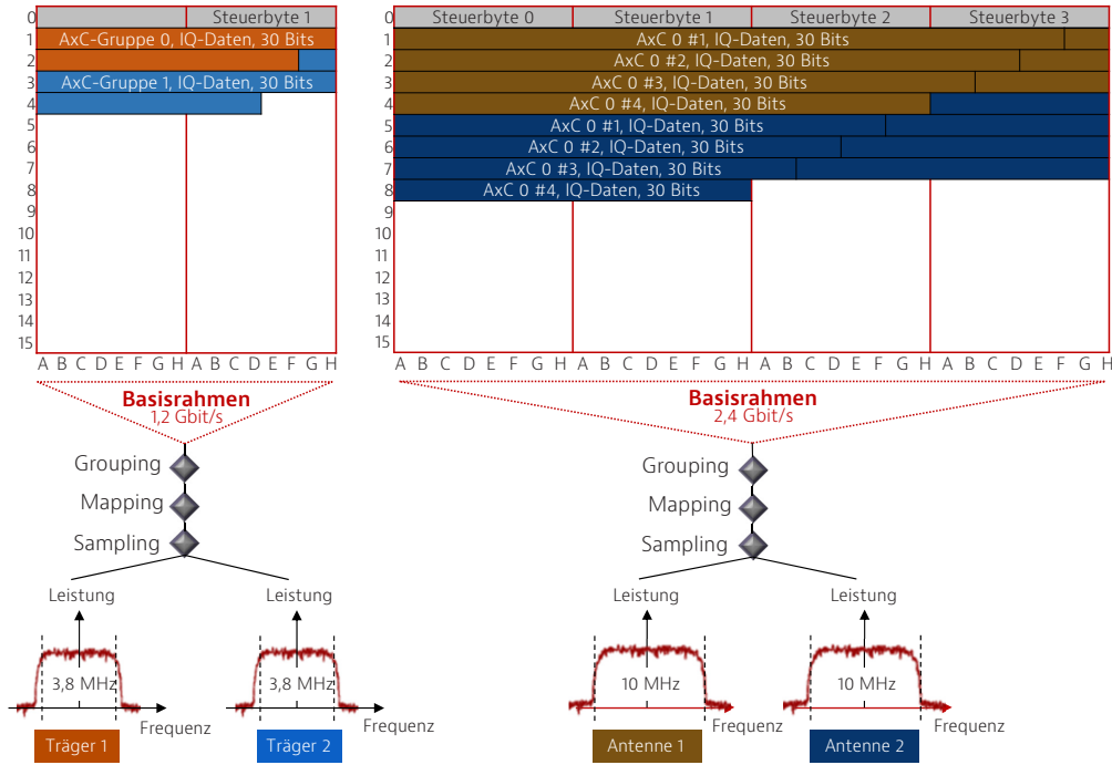
Abbildung 18: CPRI-Rahmung von UMTS-Signalen
