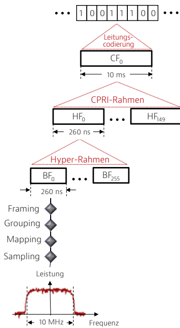
Abbildung 20: Der CPRI-Rahmen
