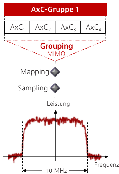
Abbildung 16: Dicht gepackte Gruppierung eines LTE-Signals von 10 MHz
