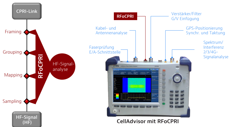
Abbildung 21: Implementierung der RFoCPRI-Technologie
