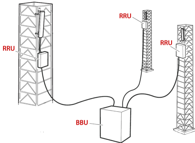
Abbildung 7: Implementierung in Baum-Topologie [5]
