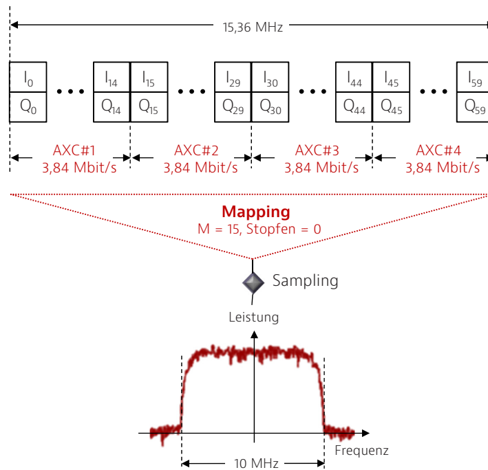
Abbildung 15: Mapping eines 10-MHz-LTE-Signals
