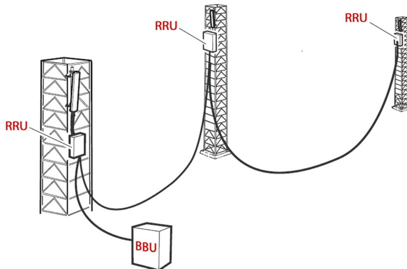
Abbildung 6: Implementierung in Ketten-Topologie [5]
