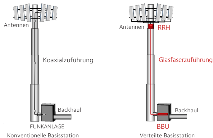
Abbildung 1: Konventionelle und verteilte Architektur von Basisstationen
