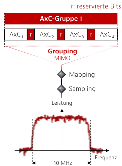
Abbildung 17: Flexible Gruppierung eines LTE-Signals von 10 MHz
