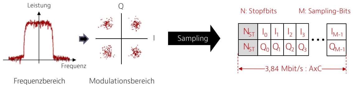
Abbildung 14: Der Abtastprozess
