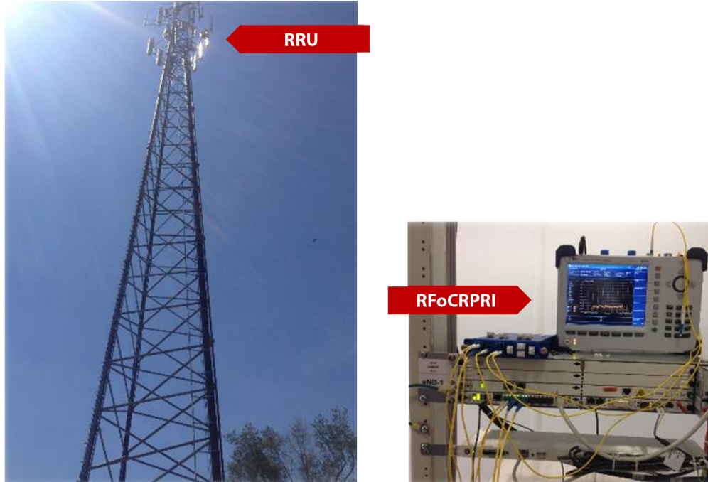
Abbildung 28: Makrozelle und CellAdvisor mit RFoCPRI
