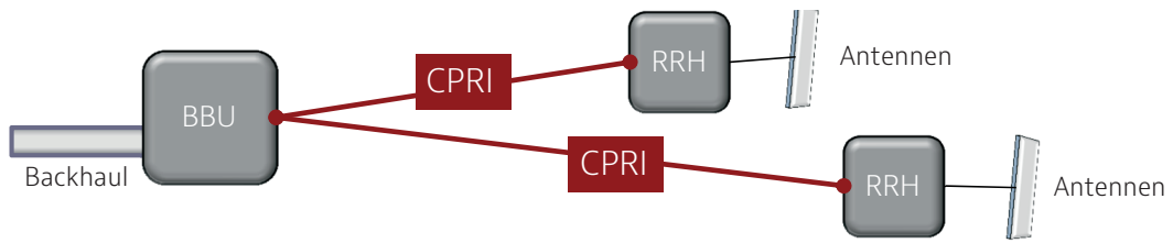
Abbildung 4: Baum-Topologie
