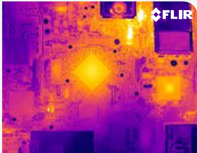
Leiterplatte
