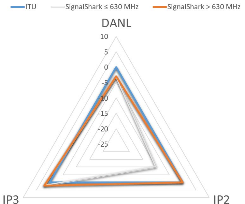
Bild 3: Dynamikparameter SignalShark im Vergleich zu den ITU
